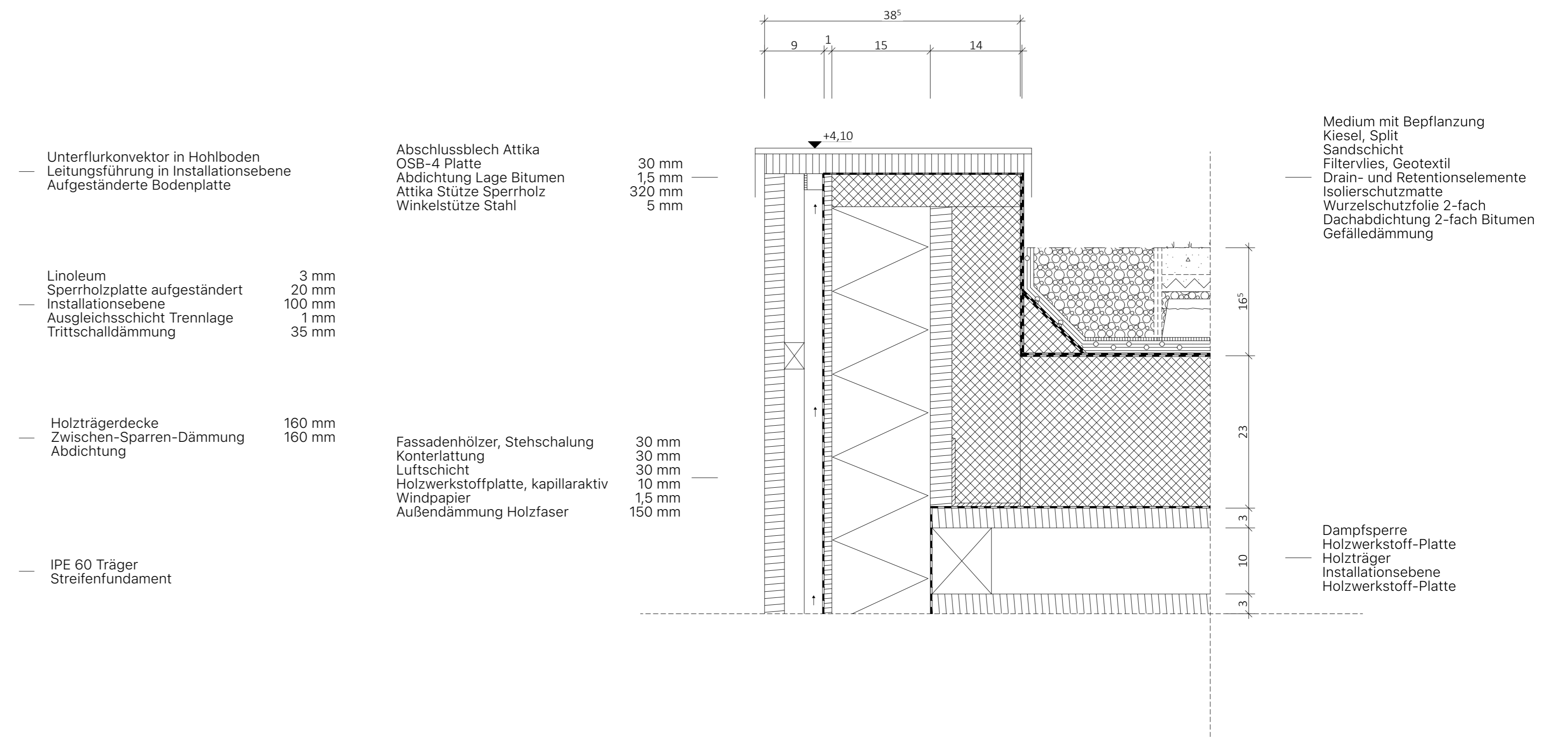
Detail Attika und Dachanschluss M 1:5
