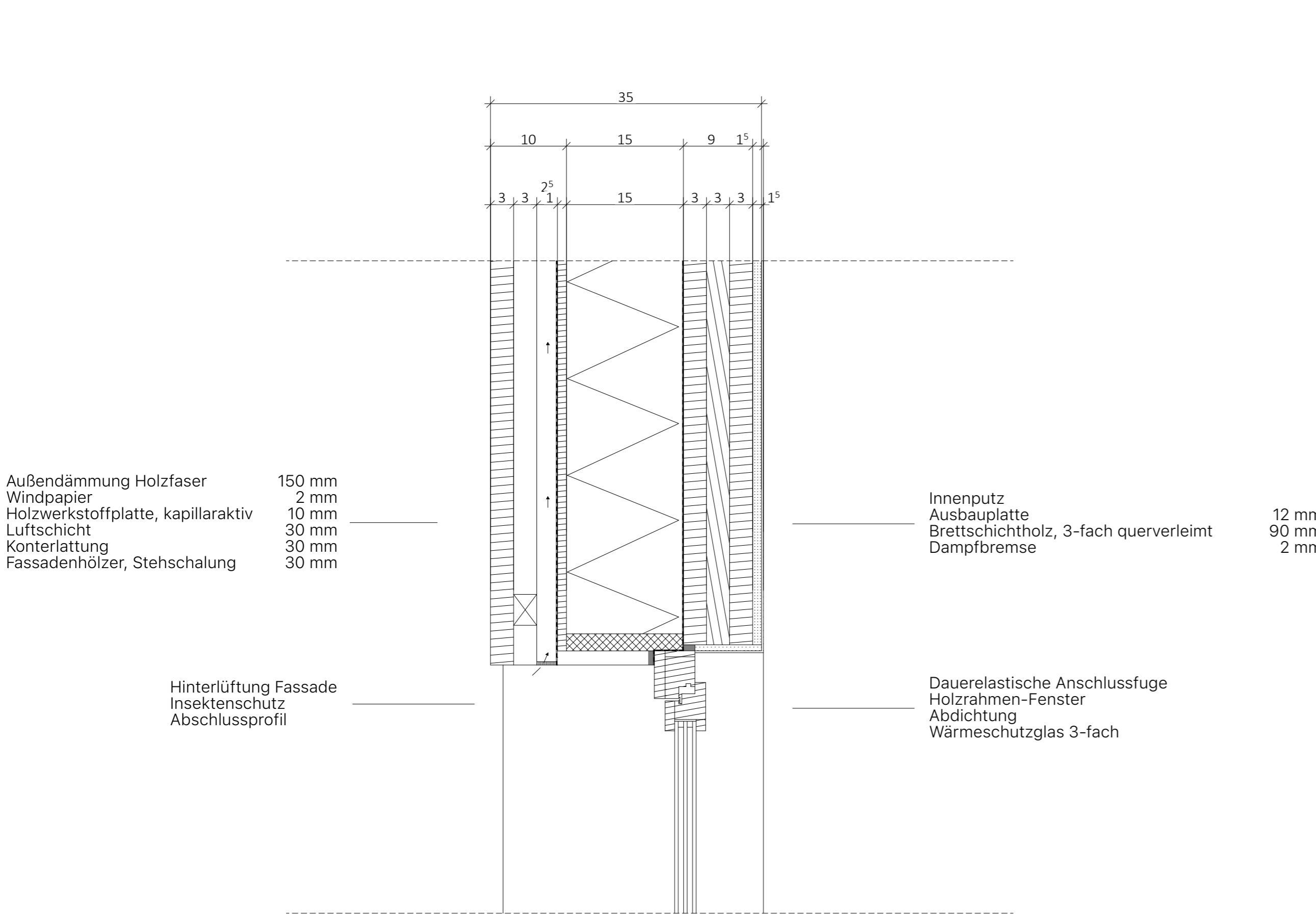
Detail Fensteranschluss M 1:5
