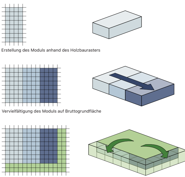
Entwurfsherleitung
