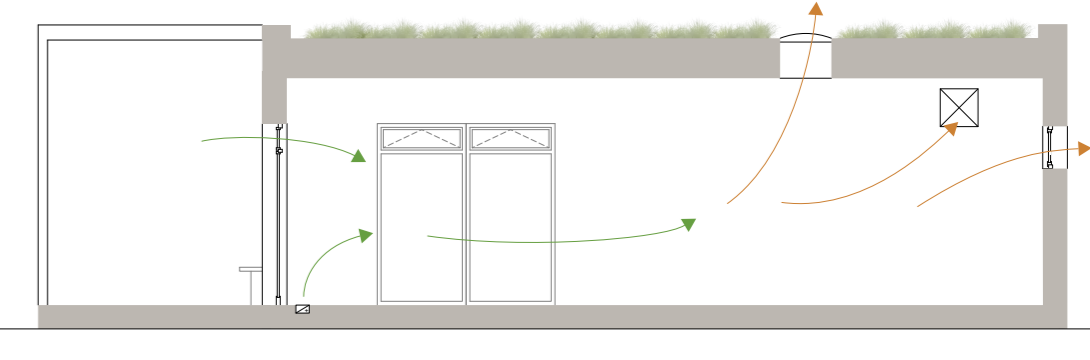
Lüftungskonzept
