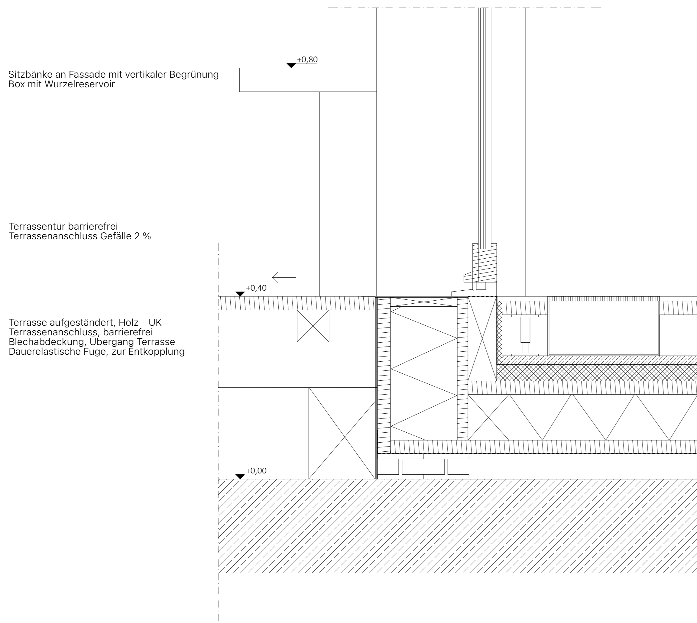
Detail Terrassenanschluss M 1:5
