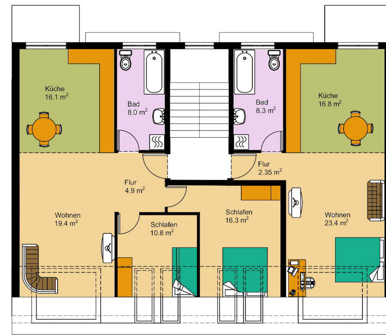
Grundriss Variante 2: 3-Zimmer-, 1-Zimmerwohnung
