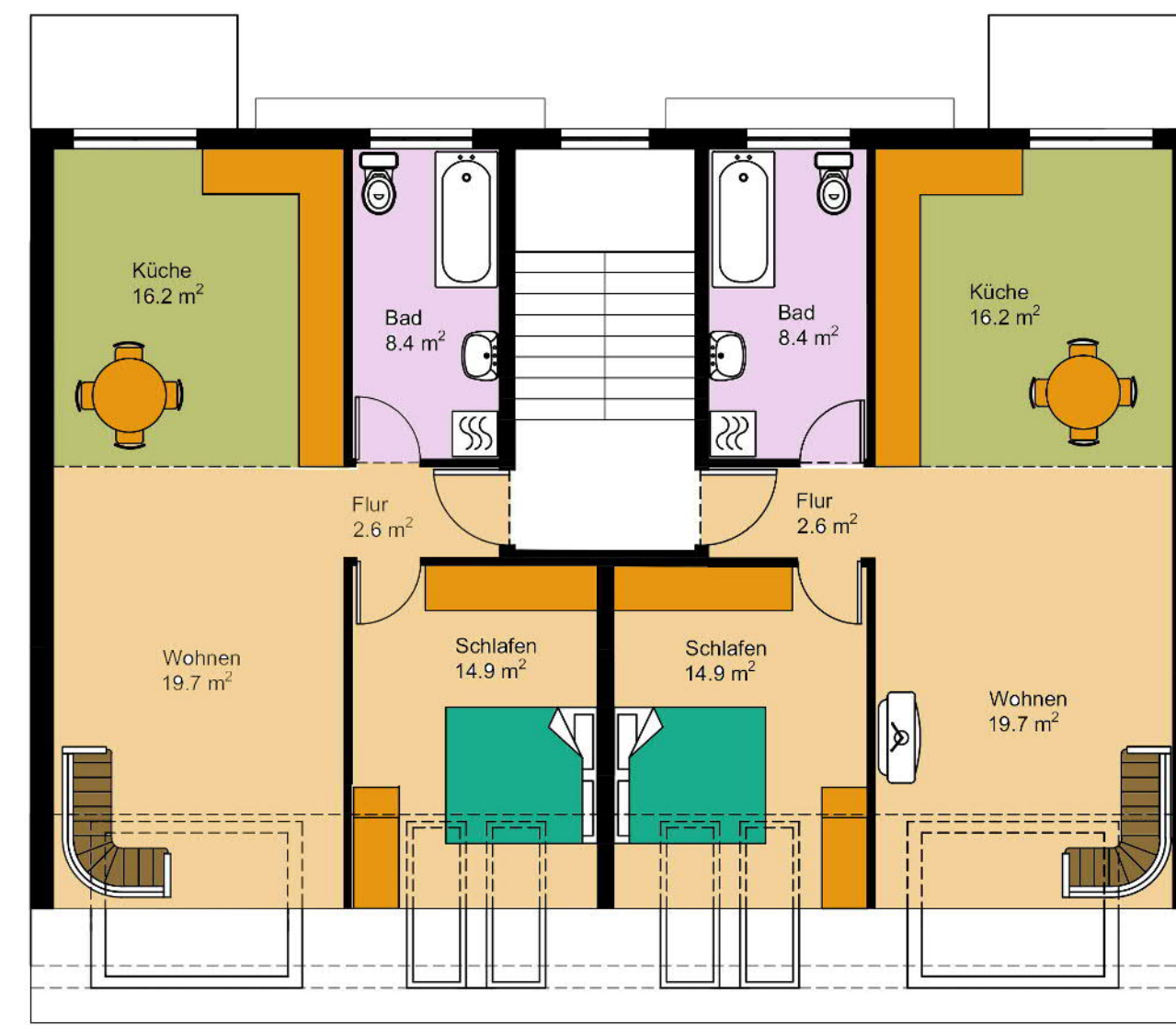
Grundriss Variante 1: 2 mal 2-Zimmerwohnung
