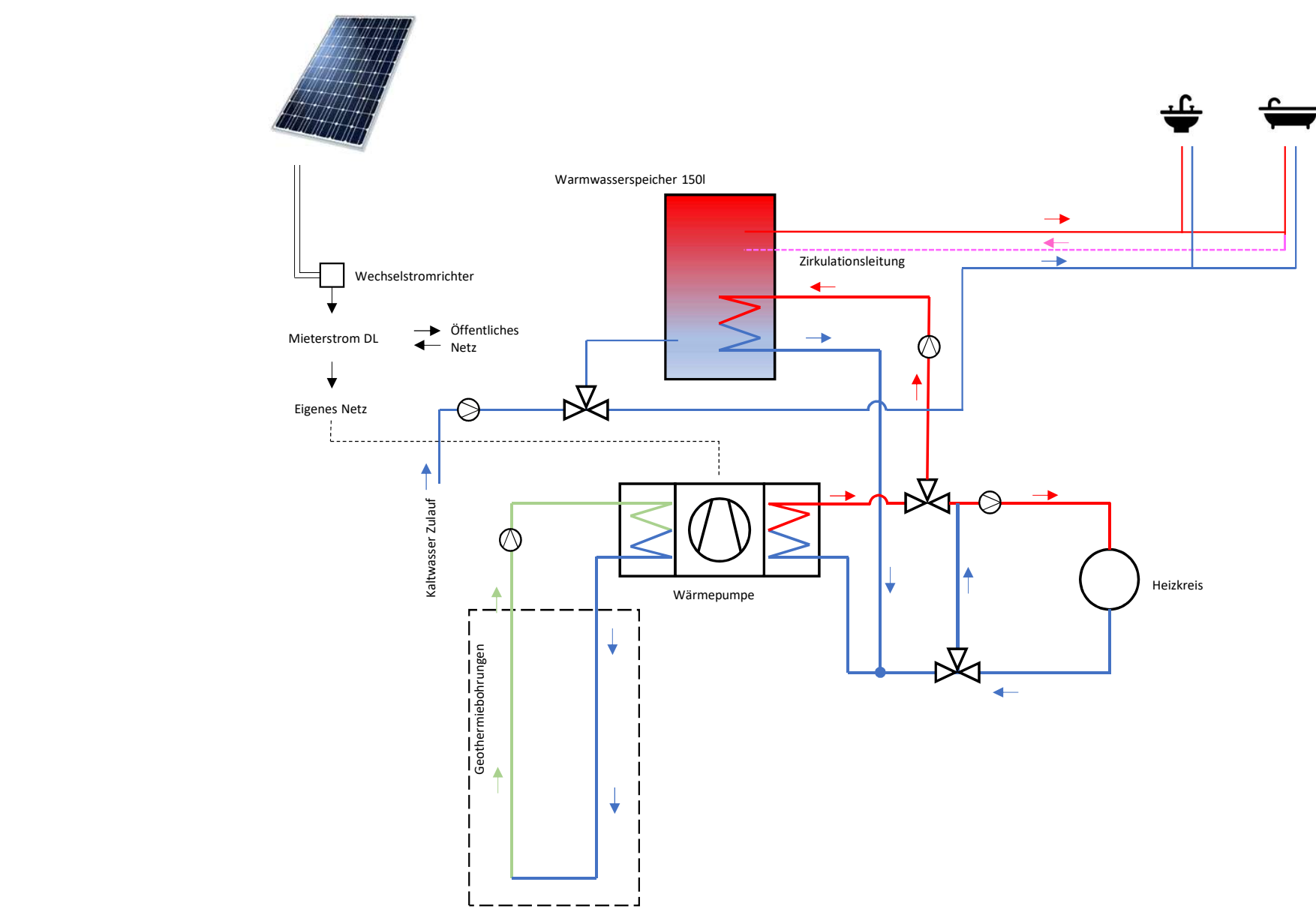
Energiekonzept
