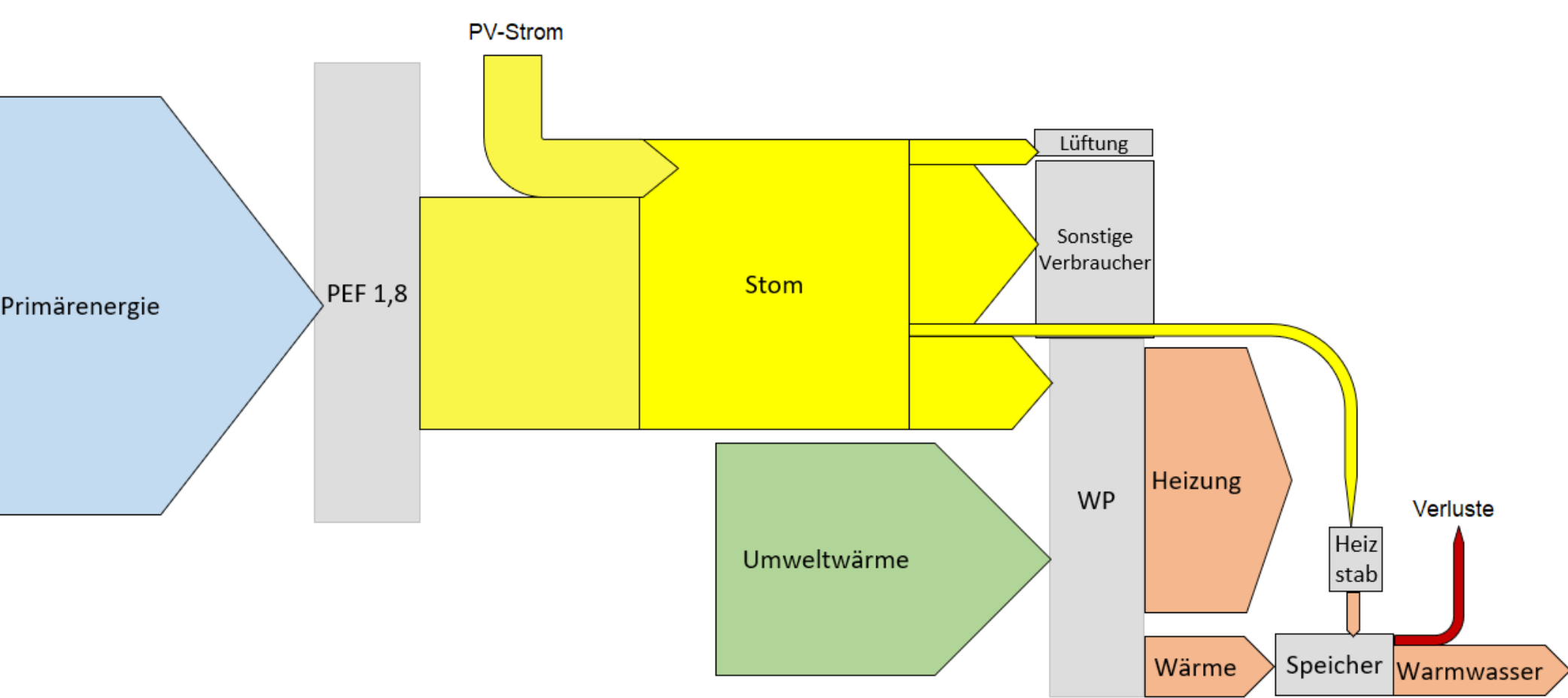
Sankey-Diagramm
