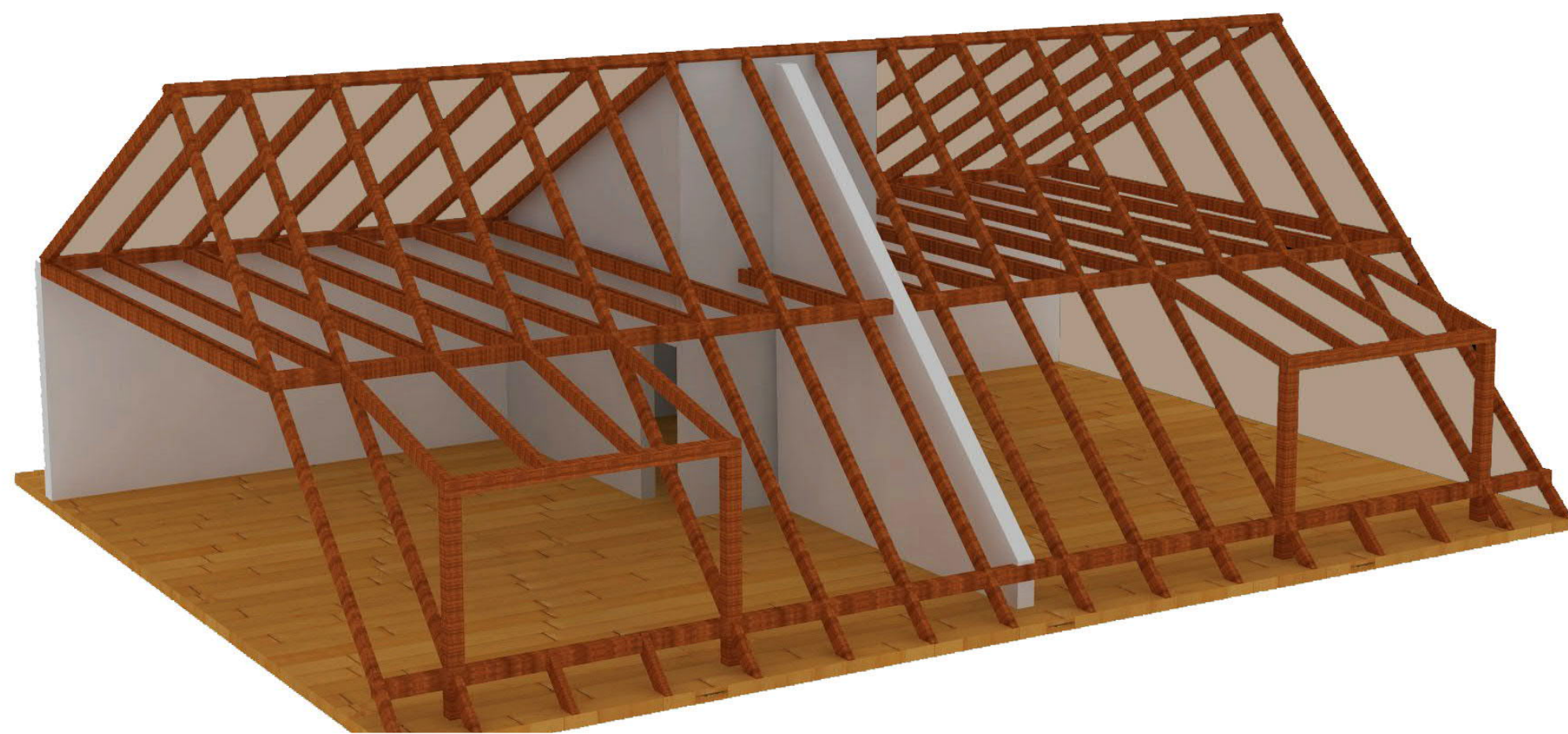
Konstruktion Dachgeschoss
